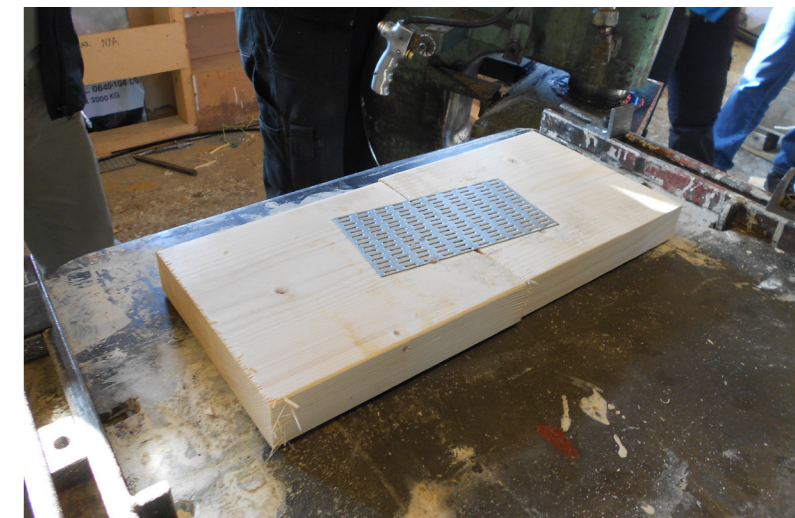
Sýnishorn af samsetningu sem notuð er á kraftsperrur
